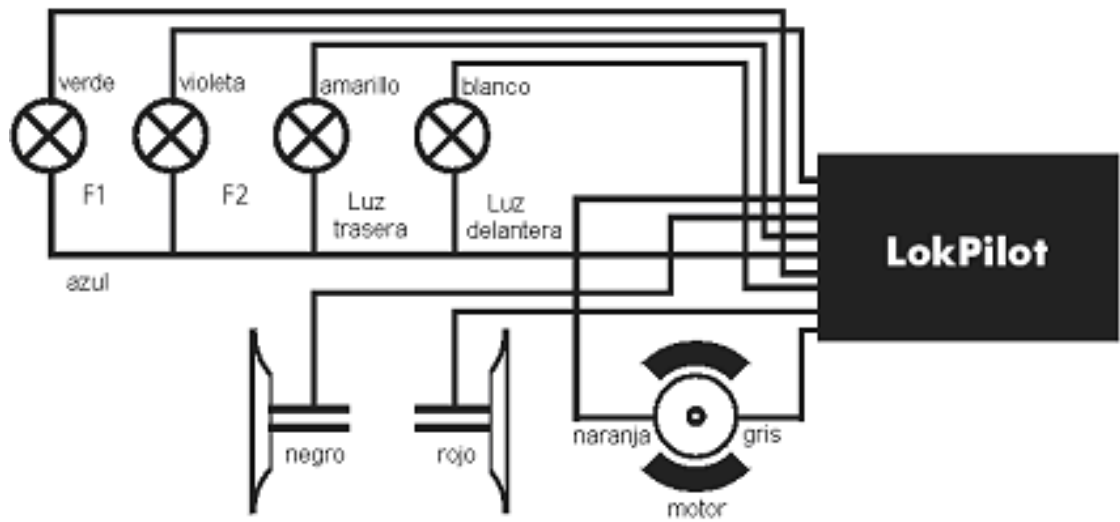
Fig. 2 – Cableado del LokPilot con funciones aislada
